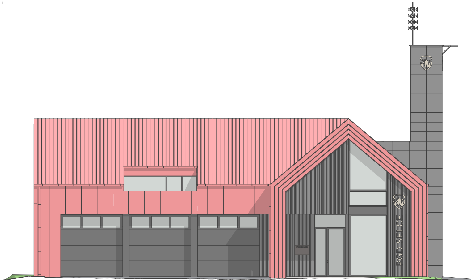
FASADA JUG
