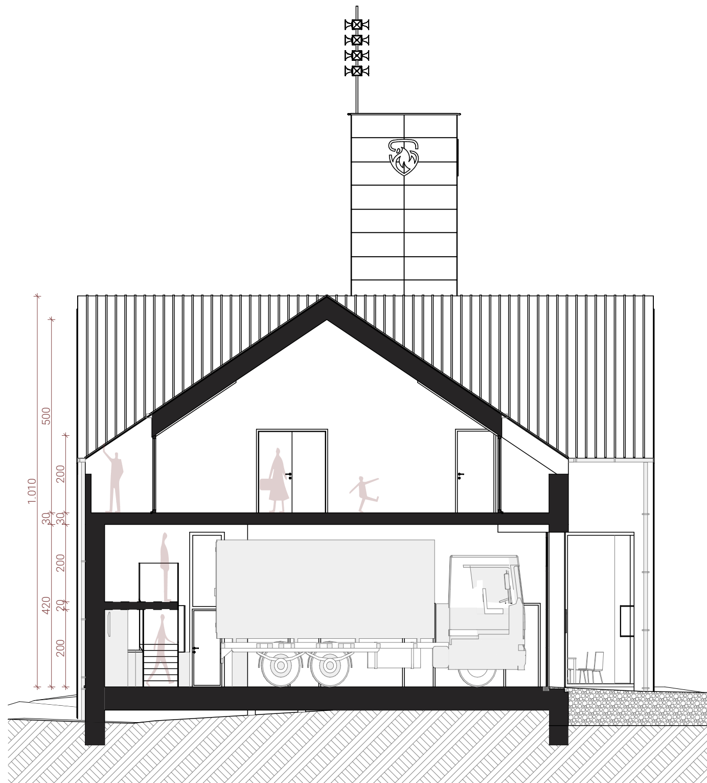
PREREZ B1
