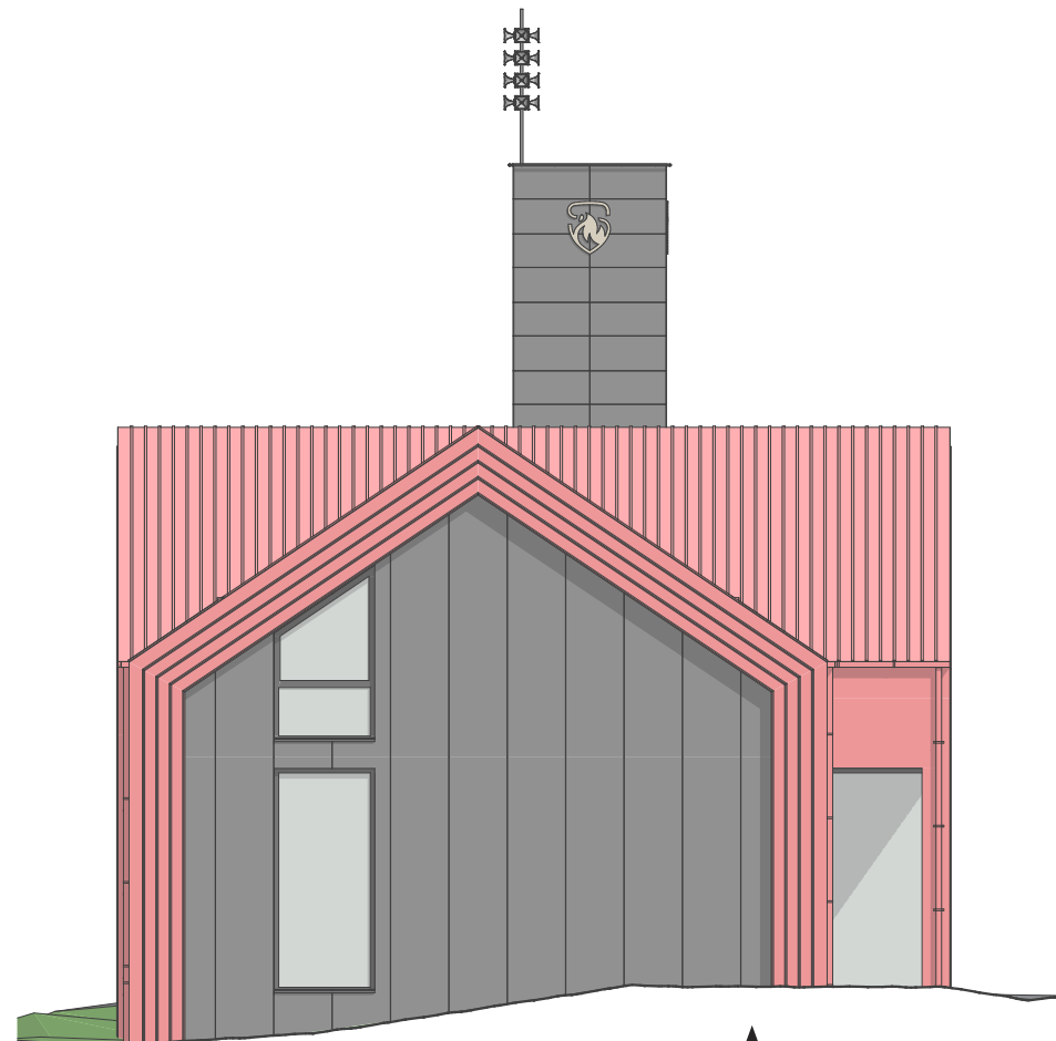
FASADA ZAHOD
